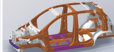
Diseño de cuerpo de jaula
